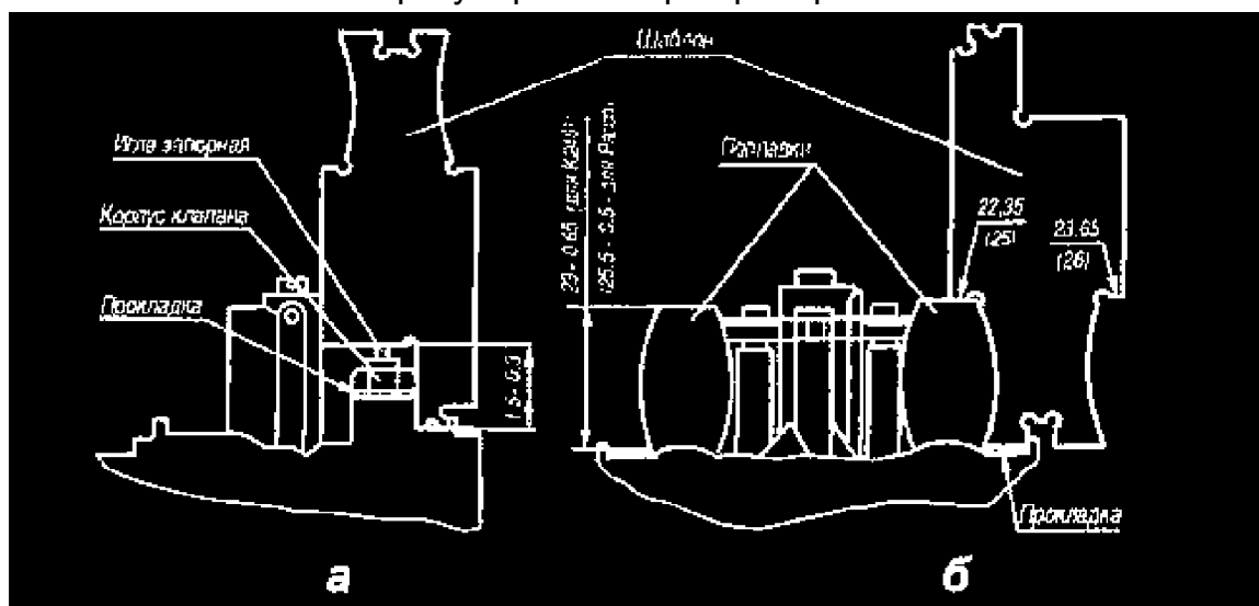
Регулировка выступаания запорной иглы клапана;
