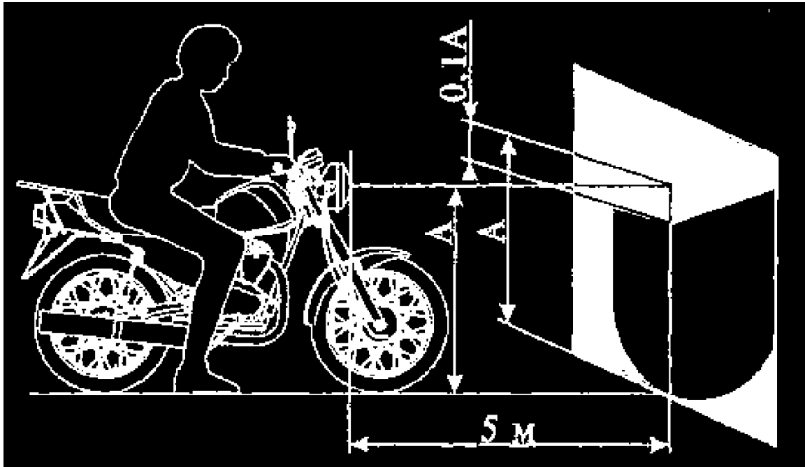
Рисунок 23 - Регулировка светового пучка фары
