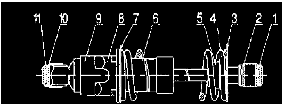
Рисунок 19а - Амортизатор гидравлический газонаполненный
