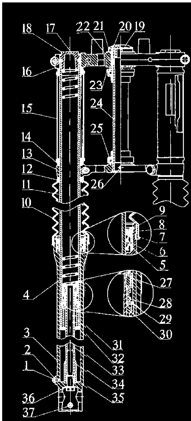
Рисунок 18 - Вилка передняя
