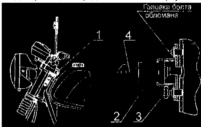
Рисунок 2б - Установка противоугонного устройства
