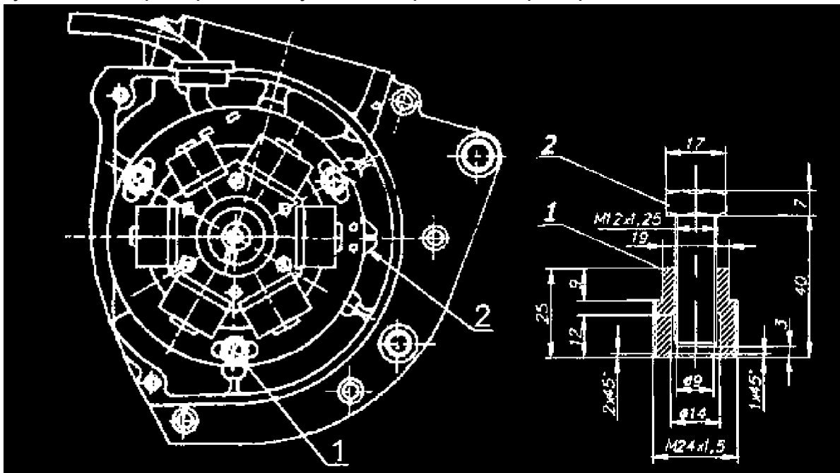
1 - съемник; 2 - болт.
