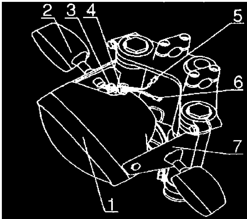
Рисунок 26 - Установка передних фонарей-указателей поворота
