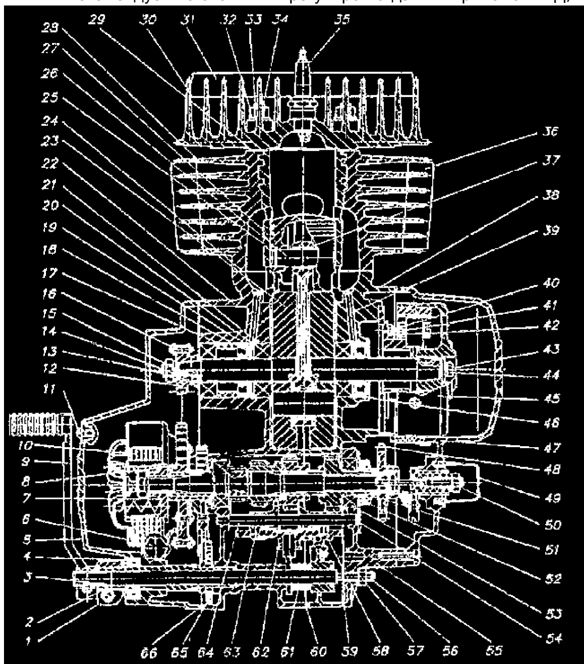
Рисунок 3 - Двигатель
