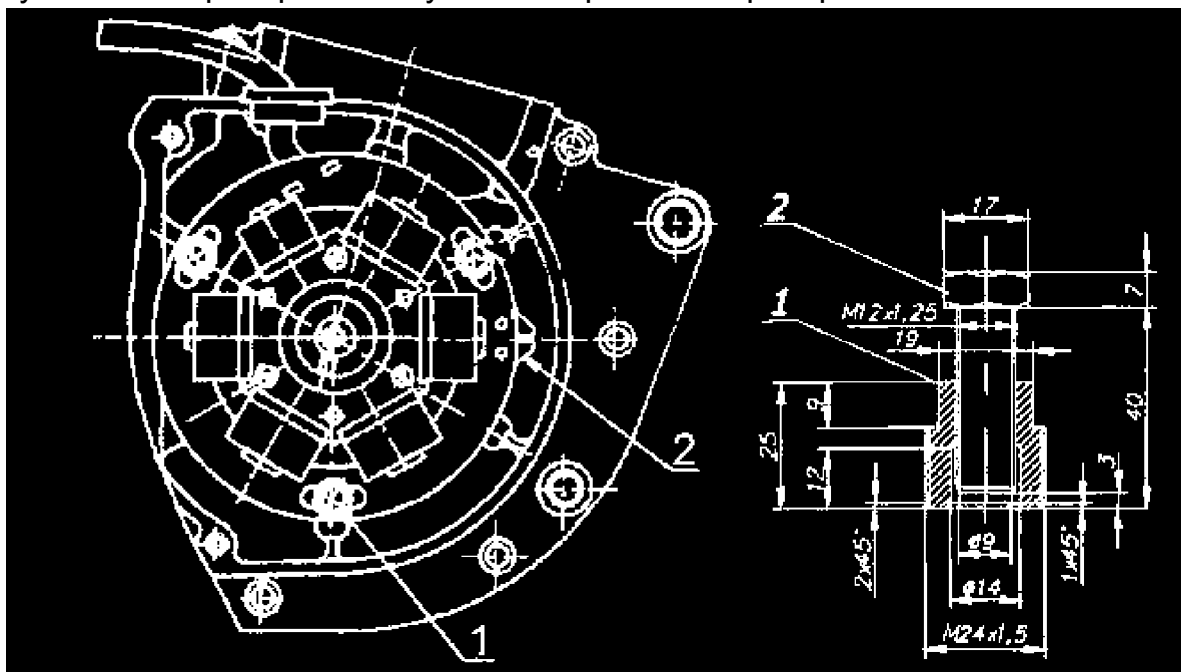
Рисунок 21 - Съемник маховичного генератора (Вид на генератор со снятым ротором)
