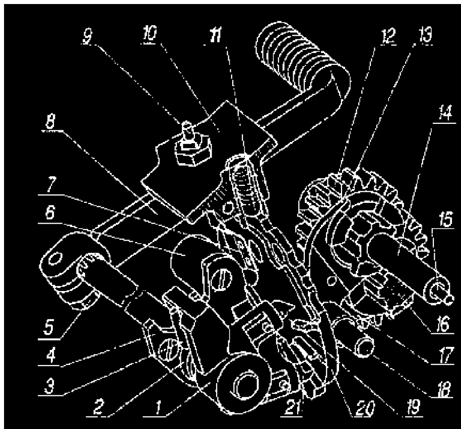
Рисунок 13 - Механизм переключения передач.
