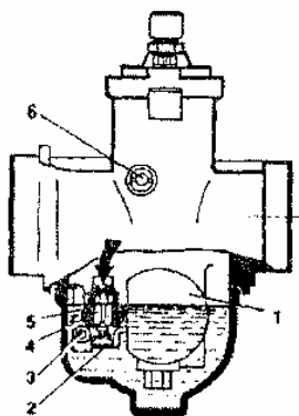
Рис.6. Поплавковый механизм 1 - поплавок; 2 - рычаг; 3 - ось; 4 - запорная игла; 5 - корпус клапана; 6 - отверстие для сообщения поплавковой камеры с атмосферой.
